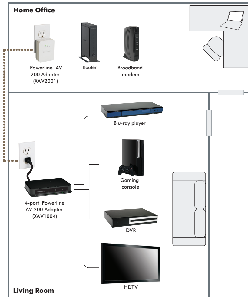
Room 2: Living Room Install the 4-port Powerline AV 200 Adapter (XAV1004)
